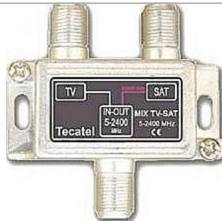
COMBINER TV-SAT
