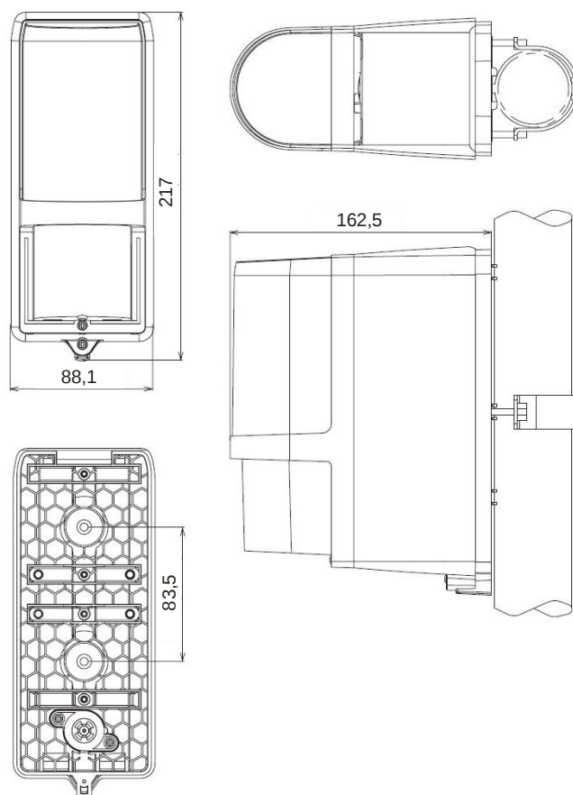
Fig. 10 Unit dimensions
